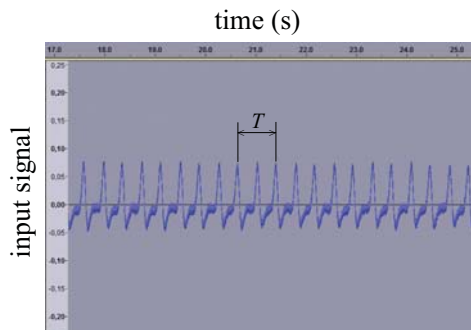
Figure 2: Pantalla de la señal eléctrica generada por el imán al oscilar dentro de una bobina de cobre. El periodo se obtiene seleccionando los tiempos en el centro de los picos señalados.
